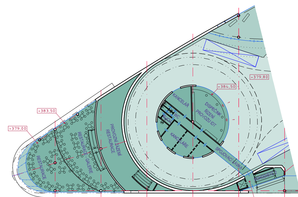
PŮDORYS 2.NP
